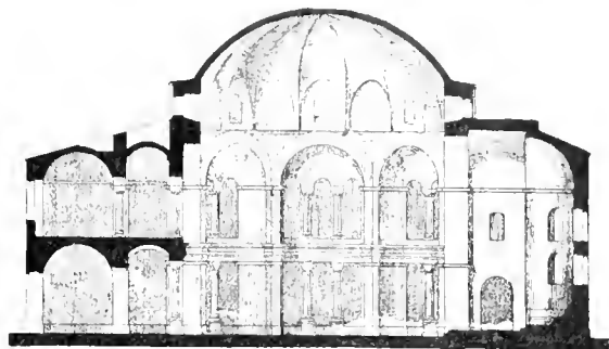
Eglise des Saints-Serge et Bacchus (coupe longitudinale).
